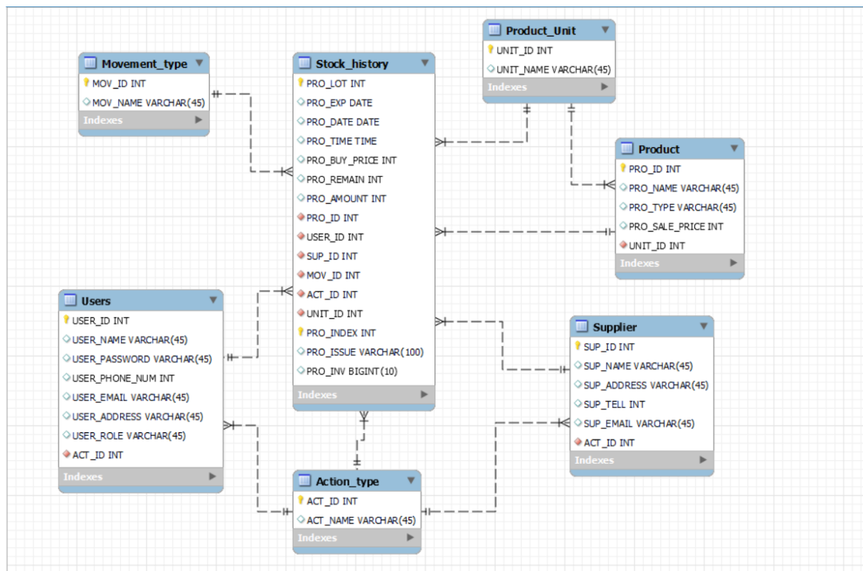
Figure 3.3 ER diagram
